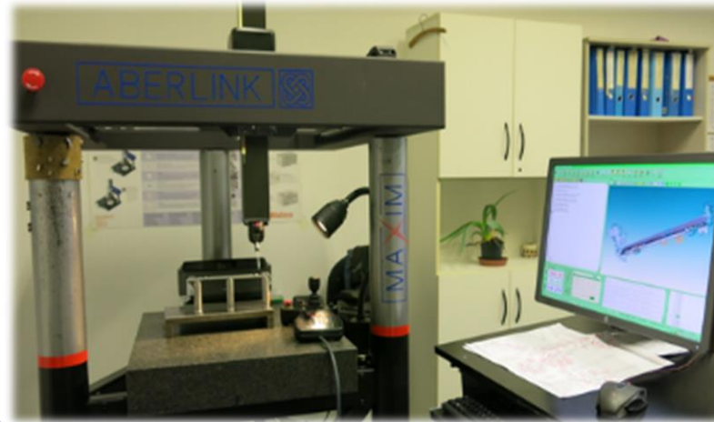
3D CNC ABERLINK MAXIM Rozsah měření 600 x 500 x 400 mm SW Renishaw MODUS
